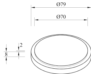
P2RH.36 Blanking Cap Trespa® HPL
